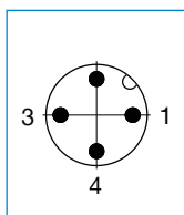
Disposición de los pines
