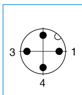
Affectation des broches
