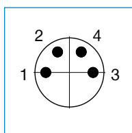
Occupazione PIN
